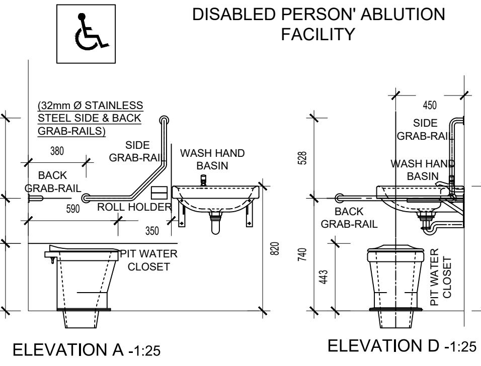
ELEVATION A -1:25
