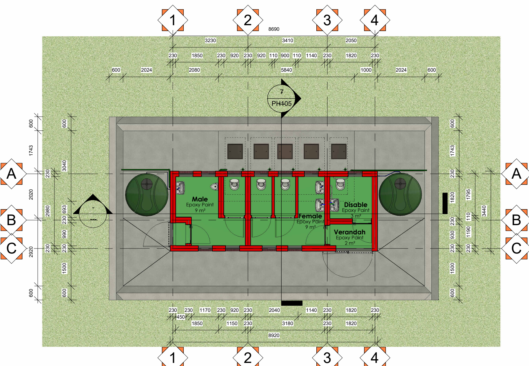
1 DWG04 Staff Toilet - Floor Plan 1 : 100
